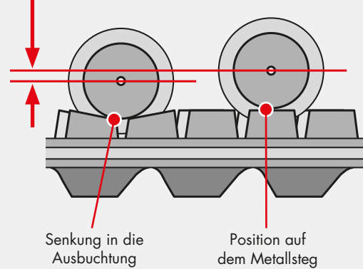
Vertikale Bewegung der Kettenrollen
