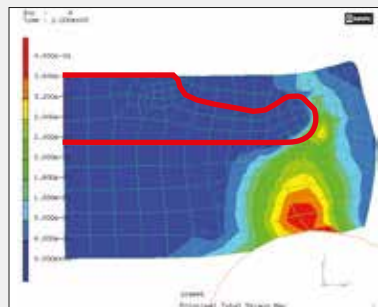
Pro-Edge Stahleinlagen
