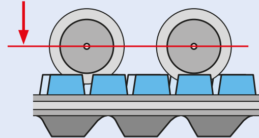
FEM Analysenergebnisse; Vertikale Bewegung der Kettenrollen
