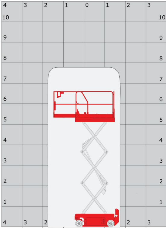
Lastdiagramm
