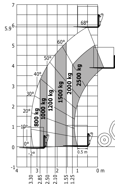
Lastdiagramm „Gelände“ (EN 1459 B)
