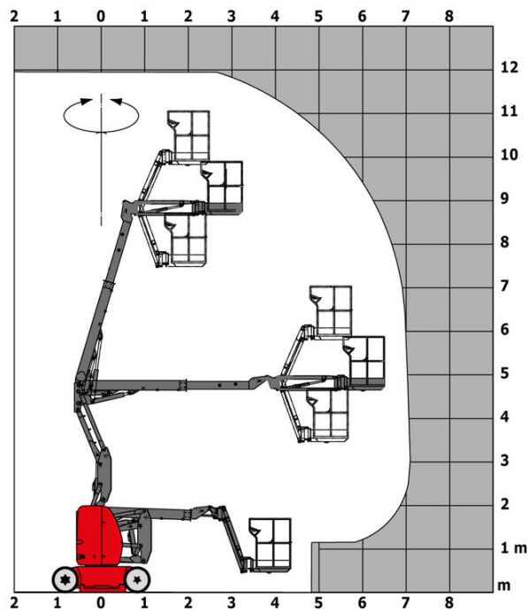
Lastdiagramm
