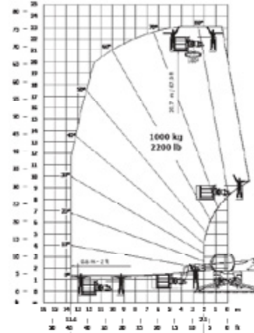
Rotierend bei ausgefahrenen Stützen mit Hubarbeitsbühne 1.000 kg EN 280
