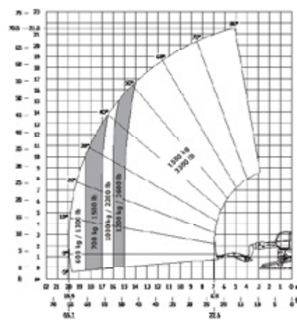
Rotierend bei ausgefahrenen Stützen mit Kranausleger 1.500 kg EN 1459
