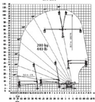
Rotierend bei ausgefahrenen Stützen Positive 3D-Arbeitsbühne EN 280
