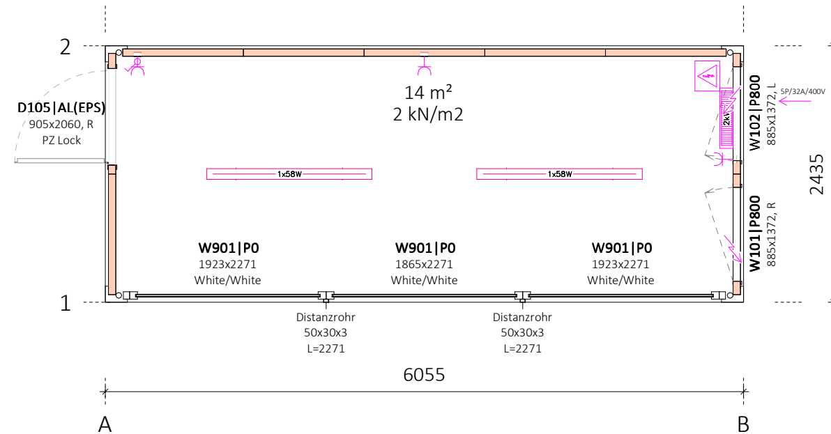
Grundriss 1 : 50
