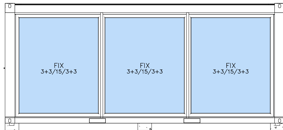
Ansicht von Vorne 1 : 50
