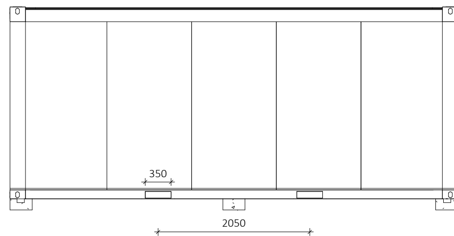
Ansicht von Rückseite 1 : 50
